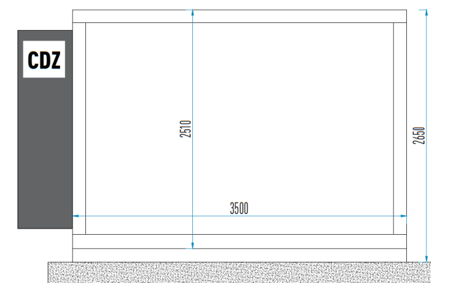
PROSPETTO FRONTALE
