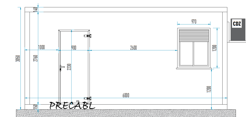
PROSPETTO FRONTALE
