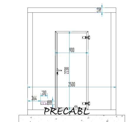
PROSPETTO LATERALE SINISTRO
