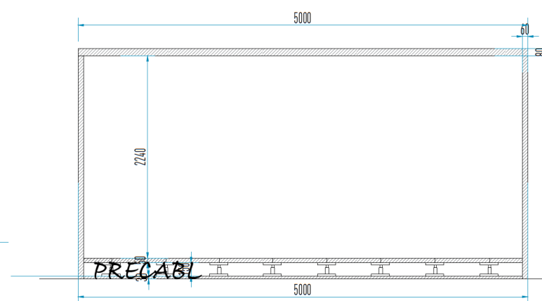
SEZIONE AA
