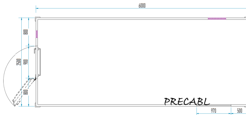
PIANTA BOX
