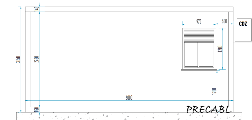
PROSPETTO FRONTALE
