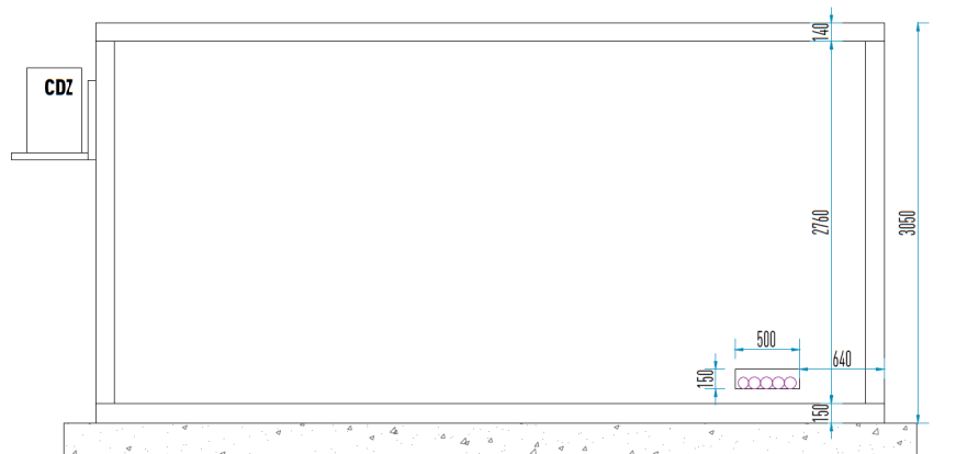
PROSPETTO POSTERIORE
