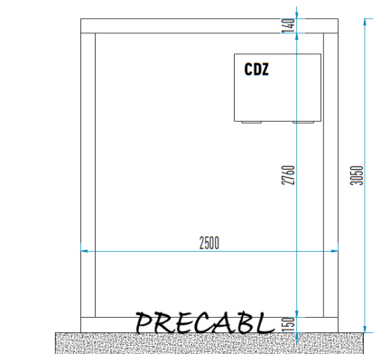
PROSPETTO LATERALE DESTRO
