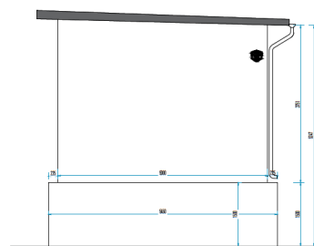
PROSPETTO LATERALE SINISTRO
