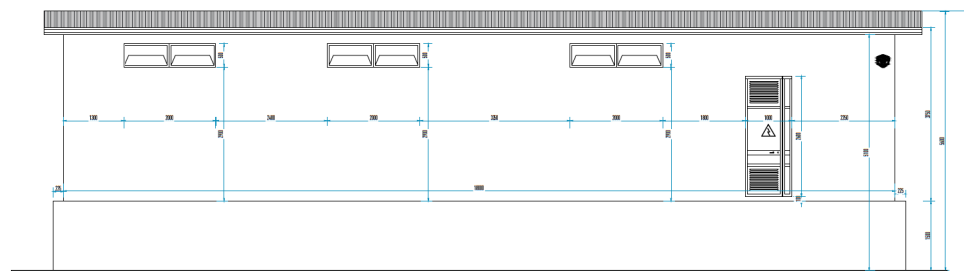
PROSPETTO POSTERIORE
