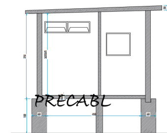
SEZIONE AA
