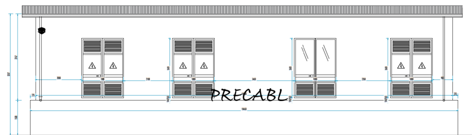
PROSPETTO ANTERIORE
