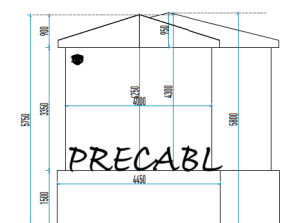
PROSPETTO LATERALE SINISTRO
