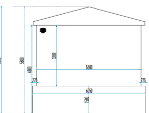
PROSPETTO LATERALE DESTRO
