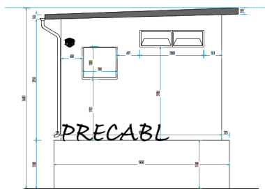
PROSPETTO LATERALE DESTRO
